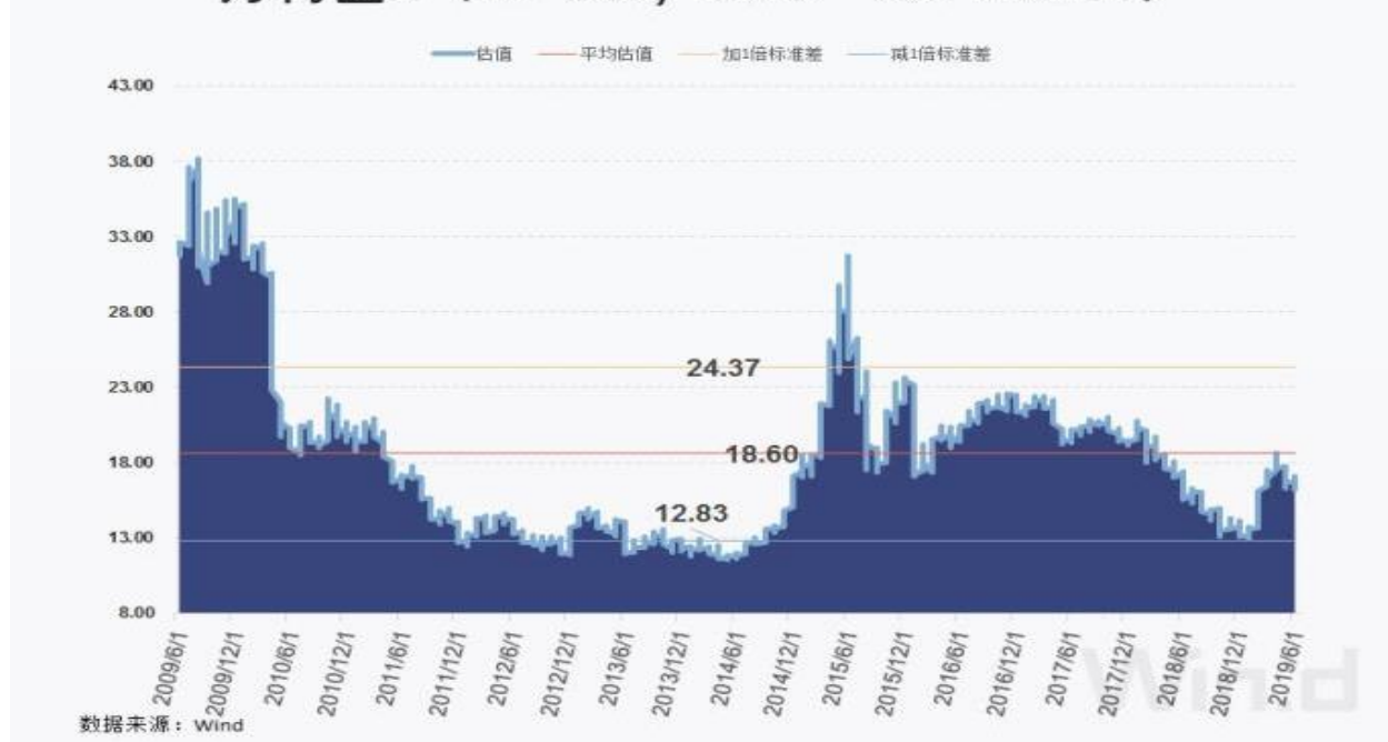
万得全A（PE-ttm, 2009—2019. 6. 21）
